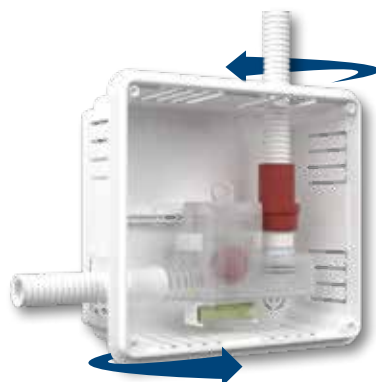
SCARICO REVERSIBILE ÉVACUATION RÉVERSIBLE REVERSIBLE OUTLET
